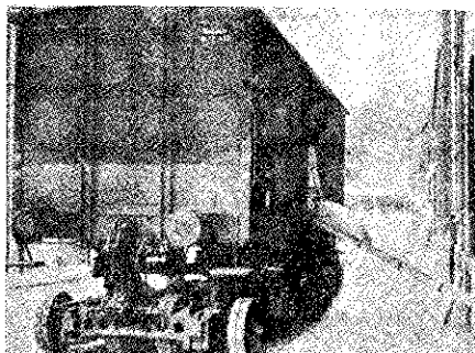
Descargando un carro ferroviario en plena calle a la puerta del comerciante gracias al dispositivo de Culemeyer. Descarga de azúcar para una firma comercial.
