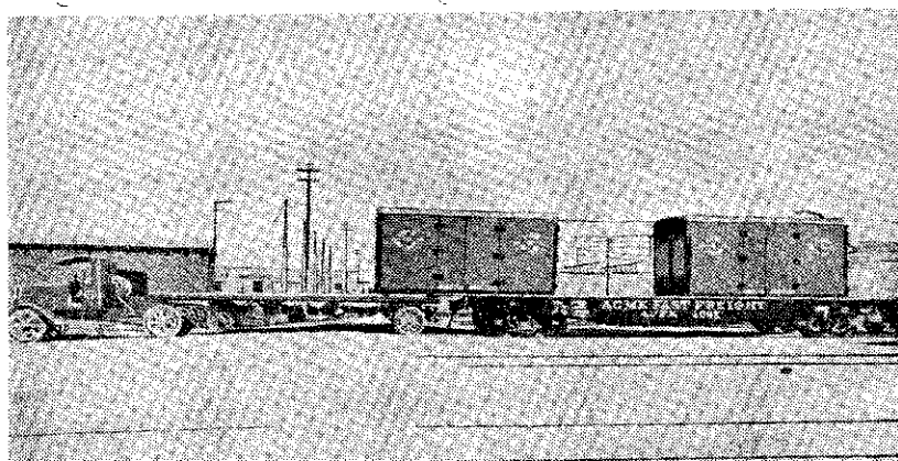
Colocando un «container» sobre un camión desde un carro plano de ferrocarril.
