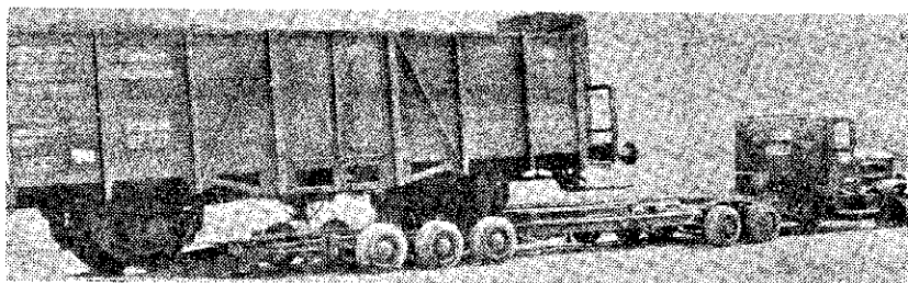
«Zorra» para el transporte de vagones ferroviarios, formando un solo vehículo con el tractor. Dispositivo mejorado, que gracias a la poca altura permite subir al vagón sobre el vehículo mediante rampa y sin necesidad de instalación especial en punta de rieles.
