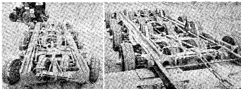
«Zorra» de 16 ruedas, para el transporte de vagones ferroviarios por calles y carreteras, ideada por el Director Culemeyer de los ferrocarriles alemanes.
